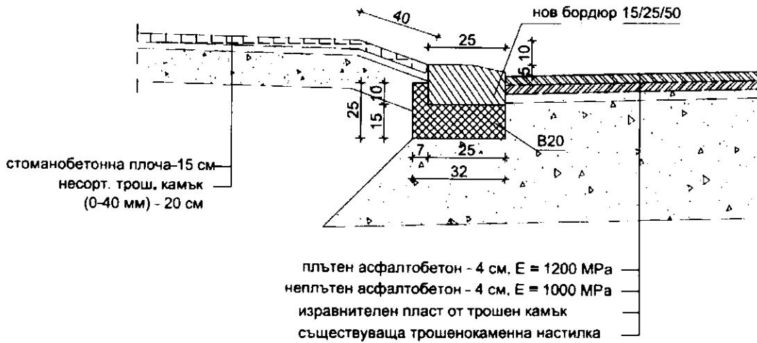
ДЕТАЙЛ ЗА ПОНИЖЕН БОРДЮР ПРЕД ВХОДОВЕ НА ГАРАЖИ М 1:20
