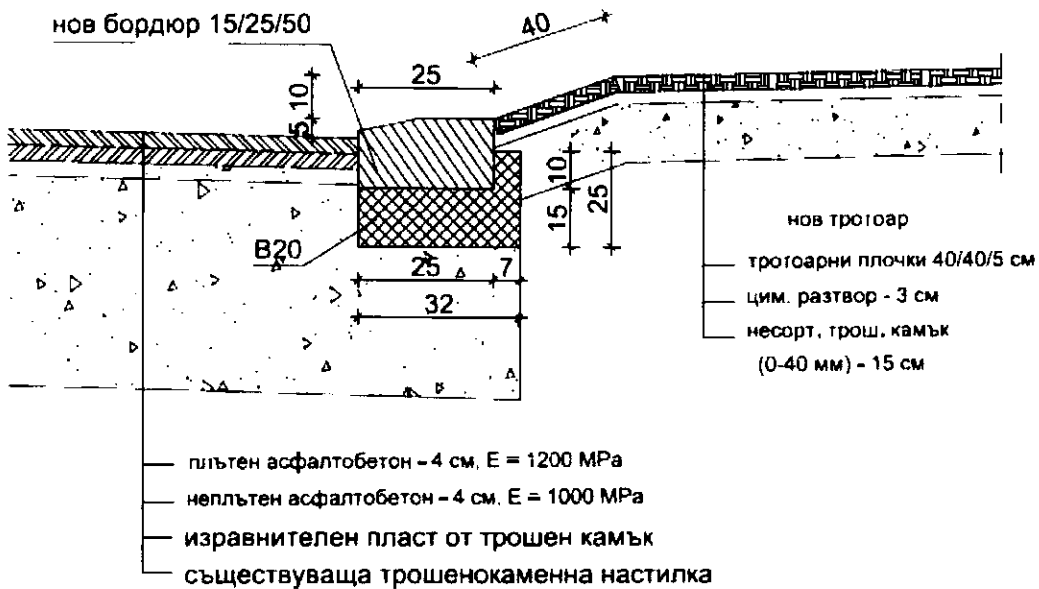
ДЕТАЙЛ ЗА ПОНИЖЕН БОРДЮР ПРЕД ВХОДОВЕ М 1:20
